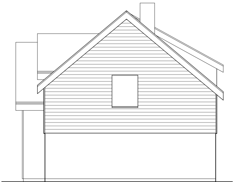
End Elevation
